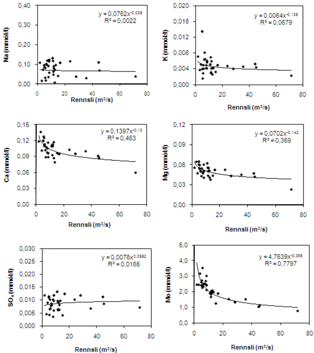
Mynd 14. Vensl styrks uppleystra aðalefna, sem rekja uppruna sinn til veðrunar bergs, við augnabliksrennsli þegar safnað var úr Norðurá við Stekk þegar sýnum var safnað á árunum 2004 til 2009.
