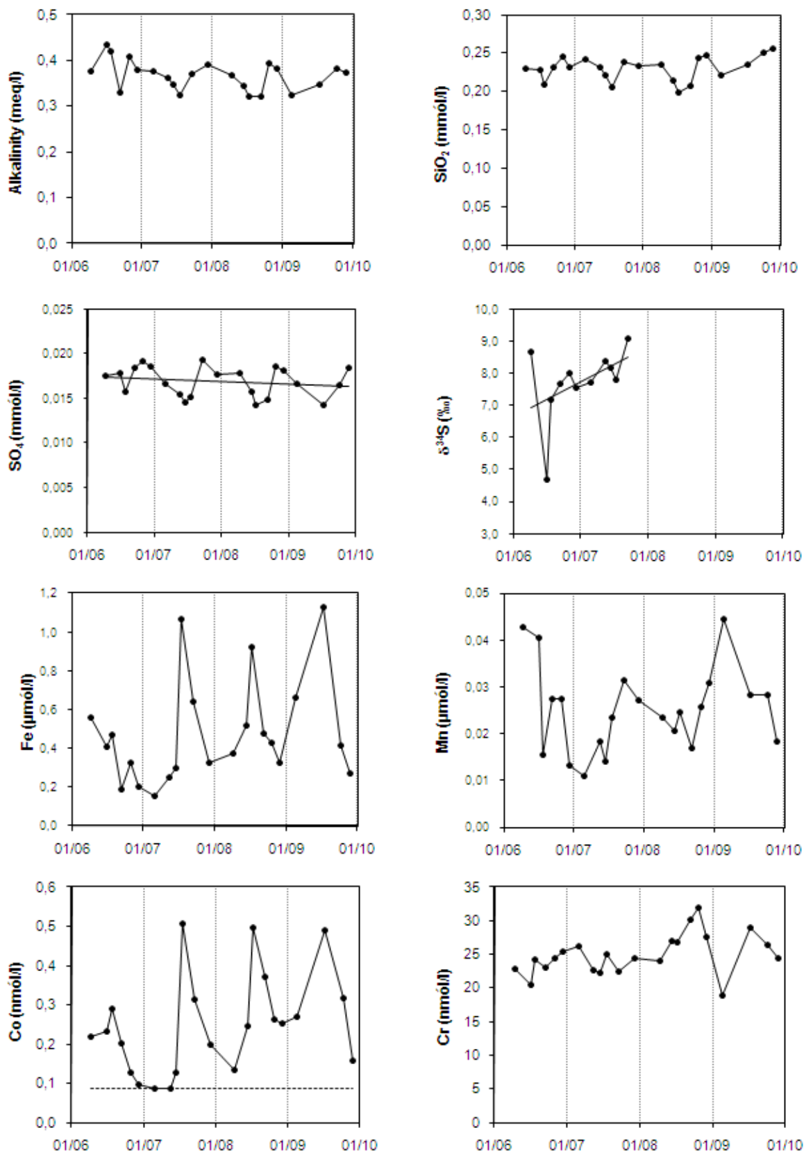
Mynd 11. Tímaraðir fyrir styrk valinna efna í Hvítá við Kljáfoss, 2006 - 2009
