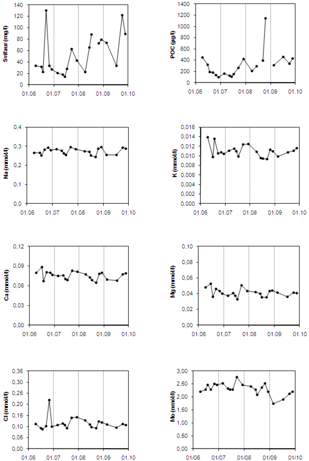
Mynd 10. Tímaraðir fyrir styrk aurburðar og valinna efna í Hvítá við Kljáfoss 2006 – 2009
