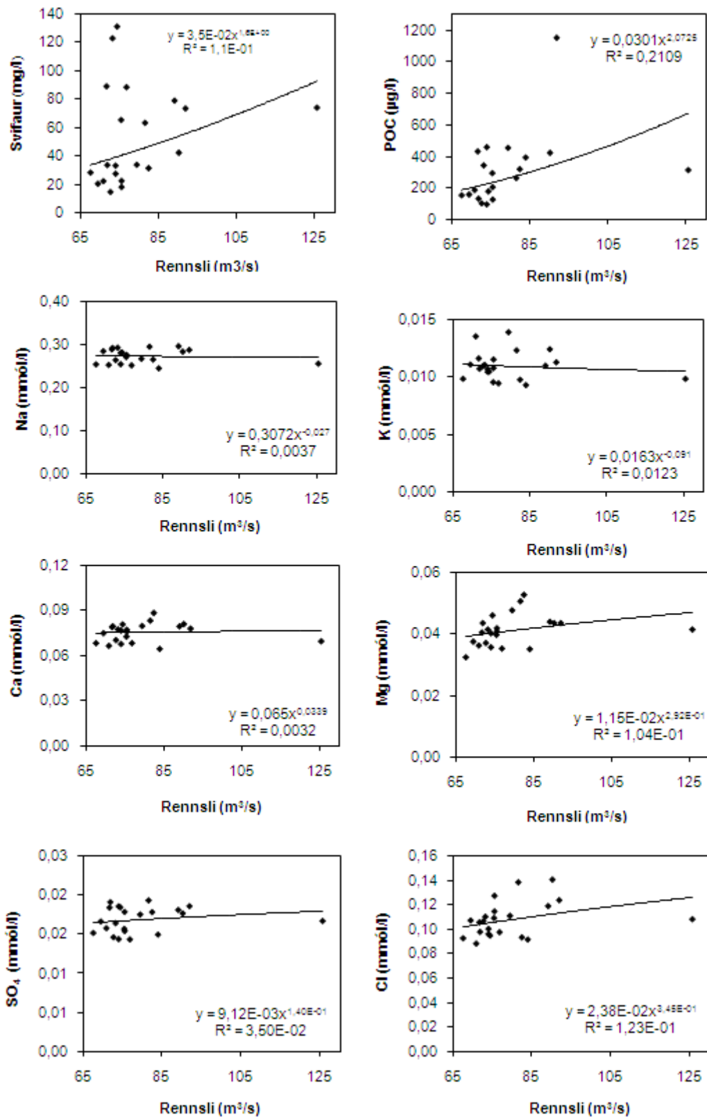
Mynd 8. Vensl augnabliksrennslis við styrk aurburðar og uppleyst aðalefni þegar sýnum var safnað úr Hvítá við Kljáfoss þegar safnað var frá 2006 til 2009.
