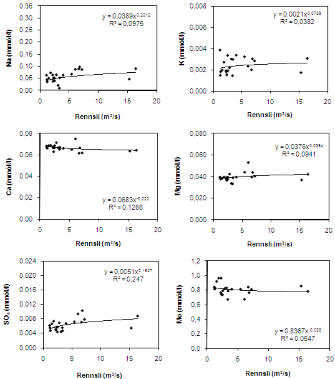
Mynd 4. Vensl styrks uppleystra aðalefna, sem rekja uppruna sinn til veðrunar bergs, við augnabliksrennsli þegar safnað var úr Andakílsá þegar sýnum var safnað frá 2006 til 2009
