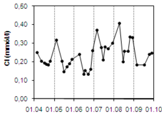
Mynd 15. Tímaraðir fyrir styrk aurburðar og valinna efna í Norðurá við Stekk 2004 – 2009.
