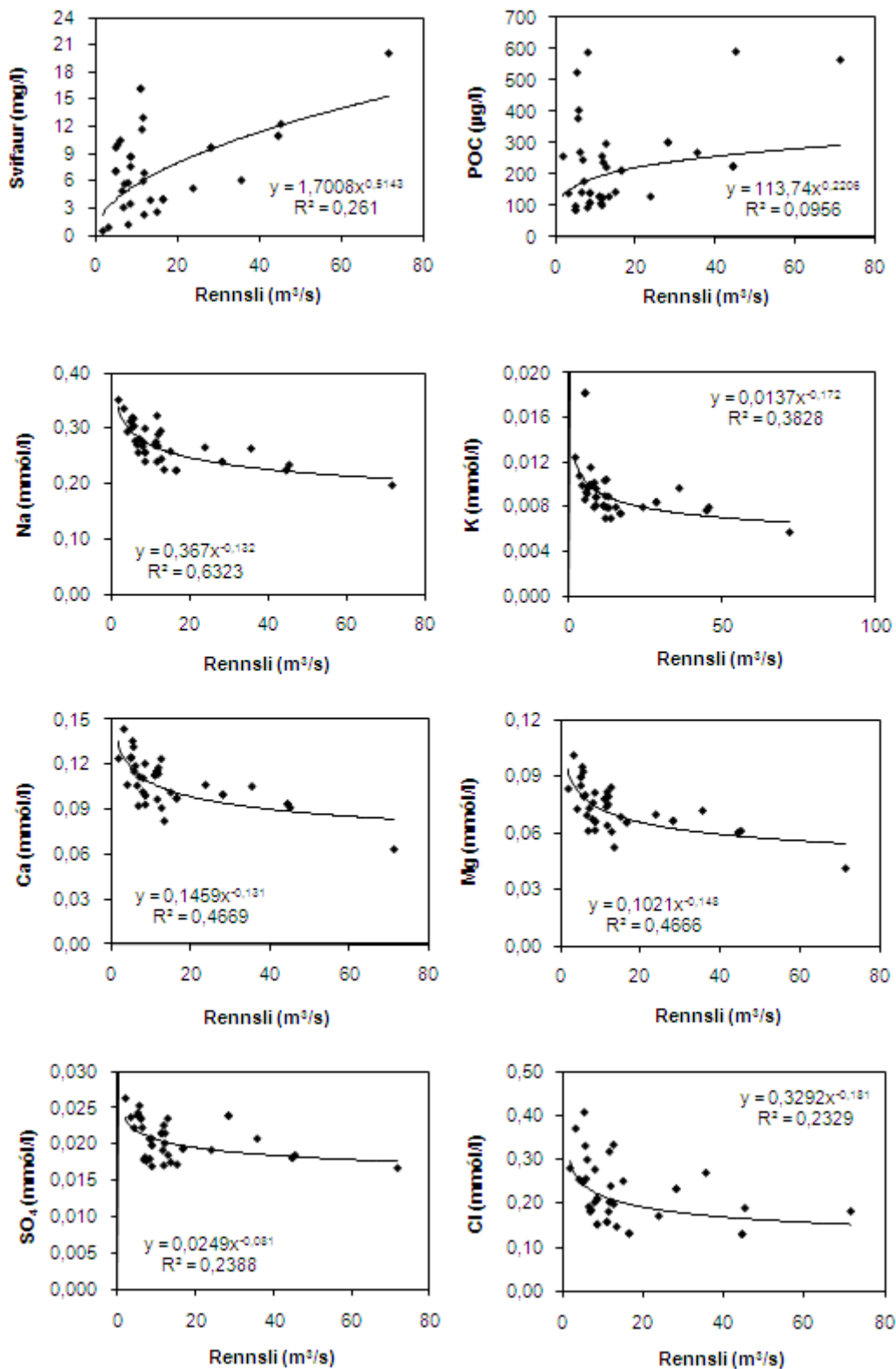
Mynd 13. Vensl augnabliksrennslið við styrk aurburðar og uppleyst aðalefni þegar safnað var úr Norðurá við Stekk þegar sýnum var safnað á árunum 2004 til 2009.
