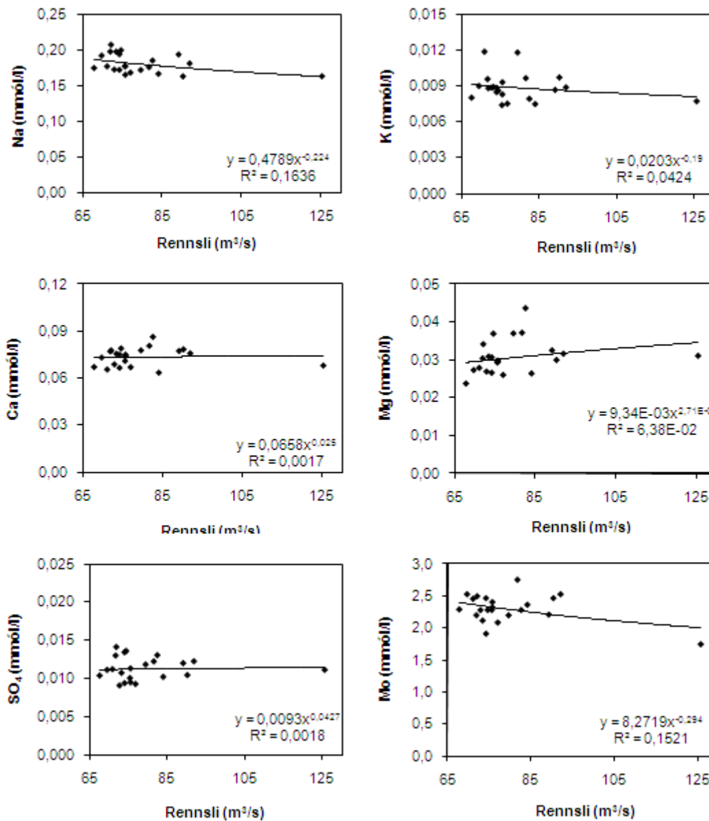
Mynd 9. Vensl styrks uppleystra aðalefna, sem rekja uppruna sinn til veðrunar bergs, við augnabliksrennsli þegar sýnum var safnað úr Hvítá við Kljáfoss frá 2006 til 2009.
