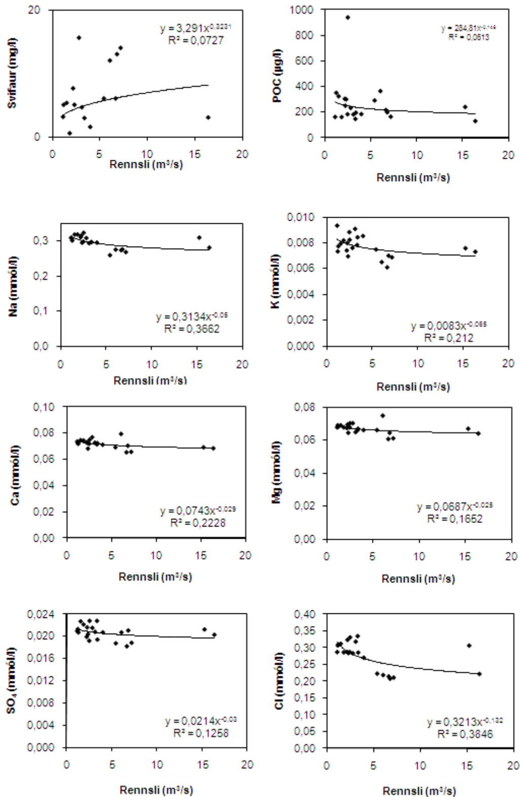
Mynd 3. Vensl augnabliksrennslis við styrk aurburðar og uppleyst aðalefni þegar safnað var úr Andakílsá þegar sýnum var safnað frá 2006-2009
