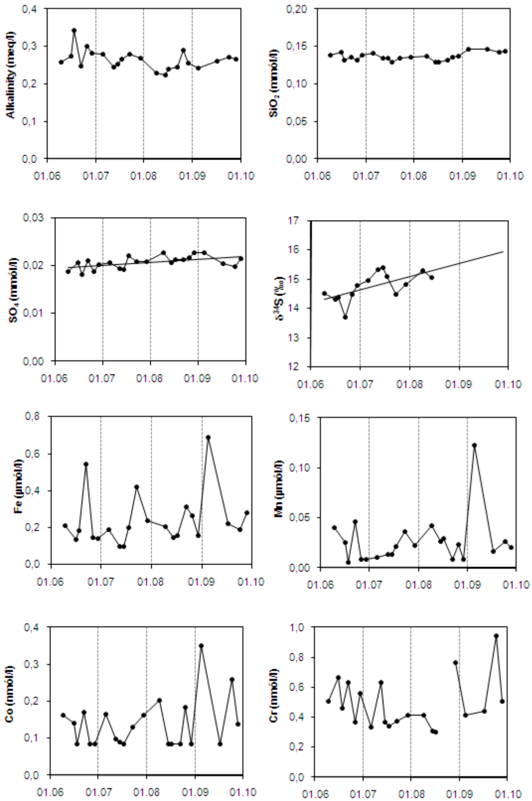
Mynd 6. Tímaraðir fyrir styrk valinna efna í Andakílsá 2006 – 2009
