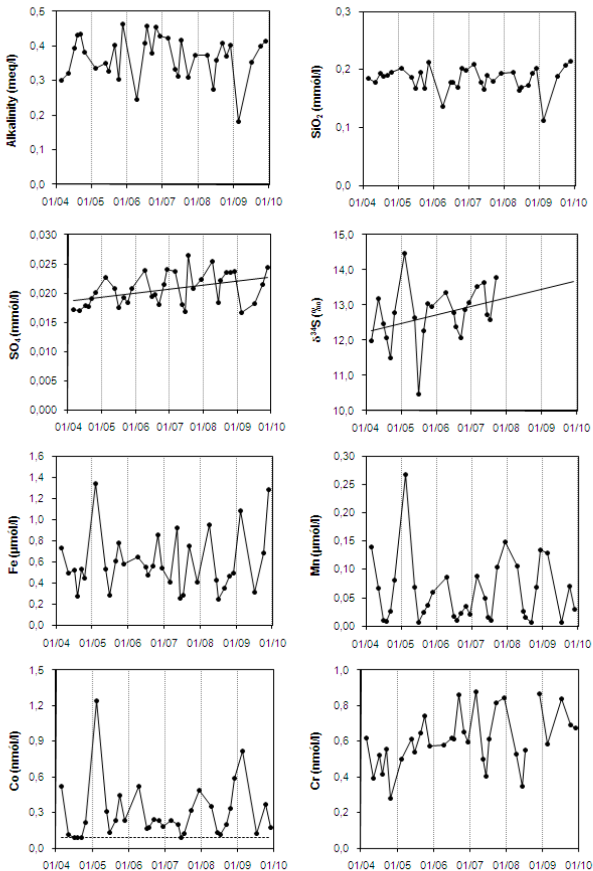
Mynd 16. Tímaraðir fyrir styrk valinna efna í Norðurá við Stekk 2004 – 2009
