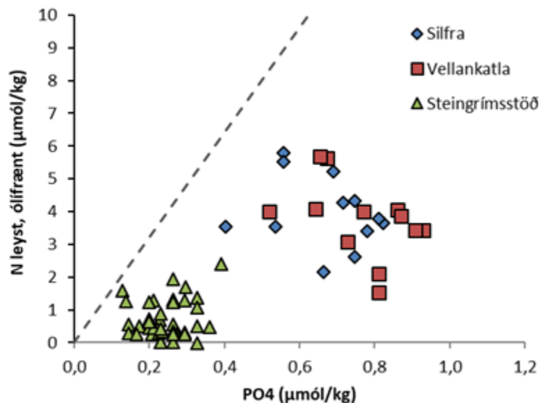
Mynd 5. Hlutföll fosfórs og niturs í inn- og útflæði Þingvallavatns eru lægri en ljóstillífandi lífverur þurfa til viðhalds. Aukning á N myndi valda aukinni þörungavirkni í vatninu. Punktalínan í myndinn sýnir mólhlutföll N/P (16/1) í þörungum.
