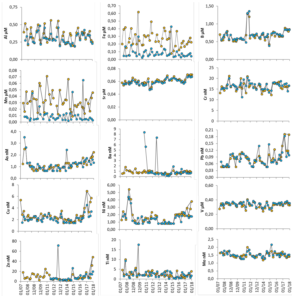
Mynd 9. Árstíðabundnar breytingar í styrk leystra snefilefna í útfalli Þingvallavatns við Steingrímsstöð og Sogi við Þrastarlund. Blár: Útfall úr Þingvallavatni við Steingrímsstöð, Gulur: Sog við Þrastarlund. Einingar eru í míkromól/l ( \mu\text{M} ) og nanómól/l (nM).
