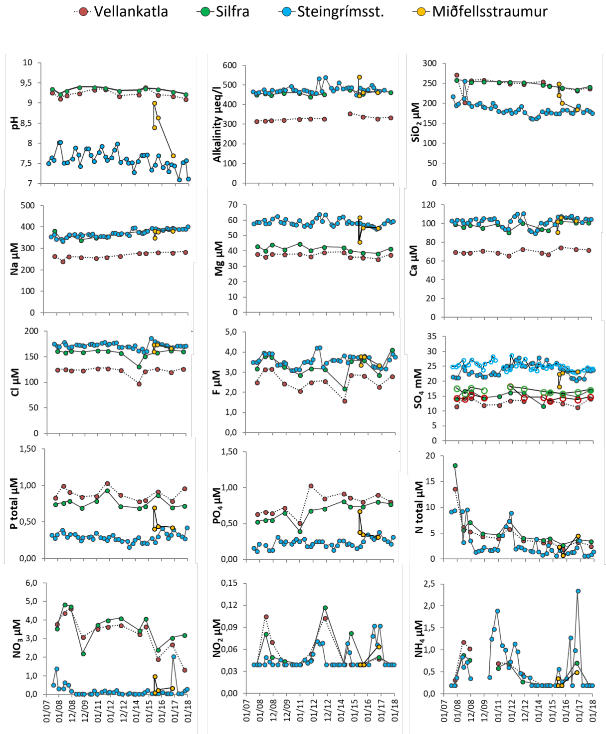
Mynd 6. Árstíðabundnar breytingar á basavirkni, pH og styrk leystra aðal- og næringarefna í inn- og útflæði Þingvallavatns. Söfnunarstaðirnir eru táknadír með mismunandi lit. Einingar eru í millimóll (mM) og míkromóll (µM).
