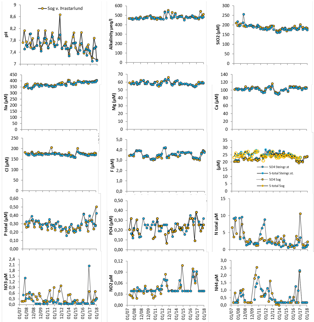
Mynd 8. Árstíðabundnar breytingar í styrk leystra aðalefna í útfalli Þingvallavatns við Steingrímsstöð og Sogi við Þrastarlund. Blár: Útfall úr Þingvallavatni við Steingrímsstöð, Gulur: Sog við Þrastarlund. Einingar eru í millimól/l (mM) og míkromól/l (µM).
