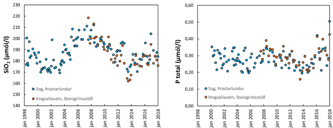
Mynd 4. Kísilstyrkur í Sogi við Þrastarlund og í útfalli Þingvallavatns við Steingrímsstöð er sveiflukennður og hefur um 10 ára sveiflutíma. Svipaða sveiflu, en ógreinilegri, má sjá í heildarstyrk fosfórs á sömu söfnunarstöðum sem bendir til breytilegrar upptöku næringarefna úr vatninu.
