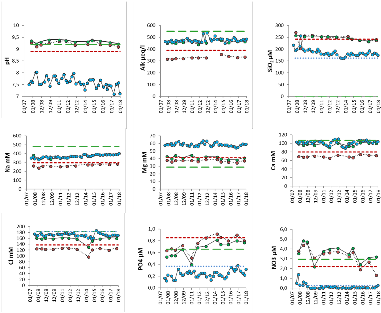
Mynd 13. Samanburður á styrk leystra efna í sýnum frá 2007-2017 við gögn sem aflað var á árunum 1975 úr Þingvallavatni og lindum sem renna í vatnið (Jón Ólafsson 1992).
