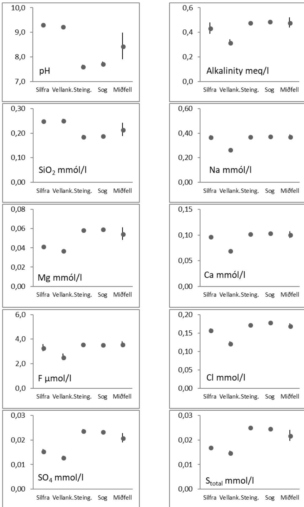
Mynd 10. Meðalstyrkur leystra aðalefna (með 95% öryggismörkum) úr innstreymi og útrennsli Þingvallavatns. Gögn úr Sogi við Þrastarlund frá 2007 til 2016 eru til samanburðar. Aðeins eru fjögur sýni úr Miðfellsstraumi.
