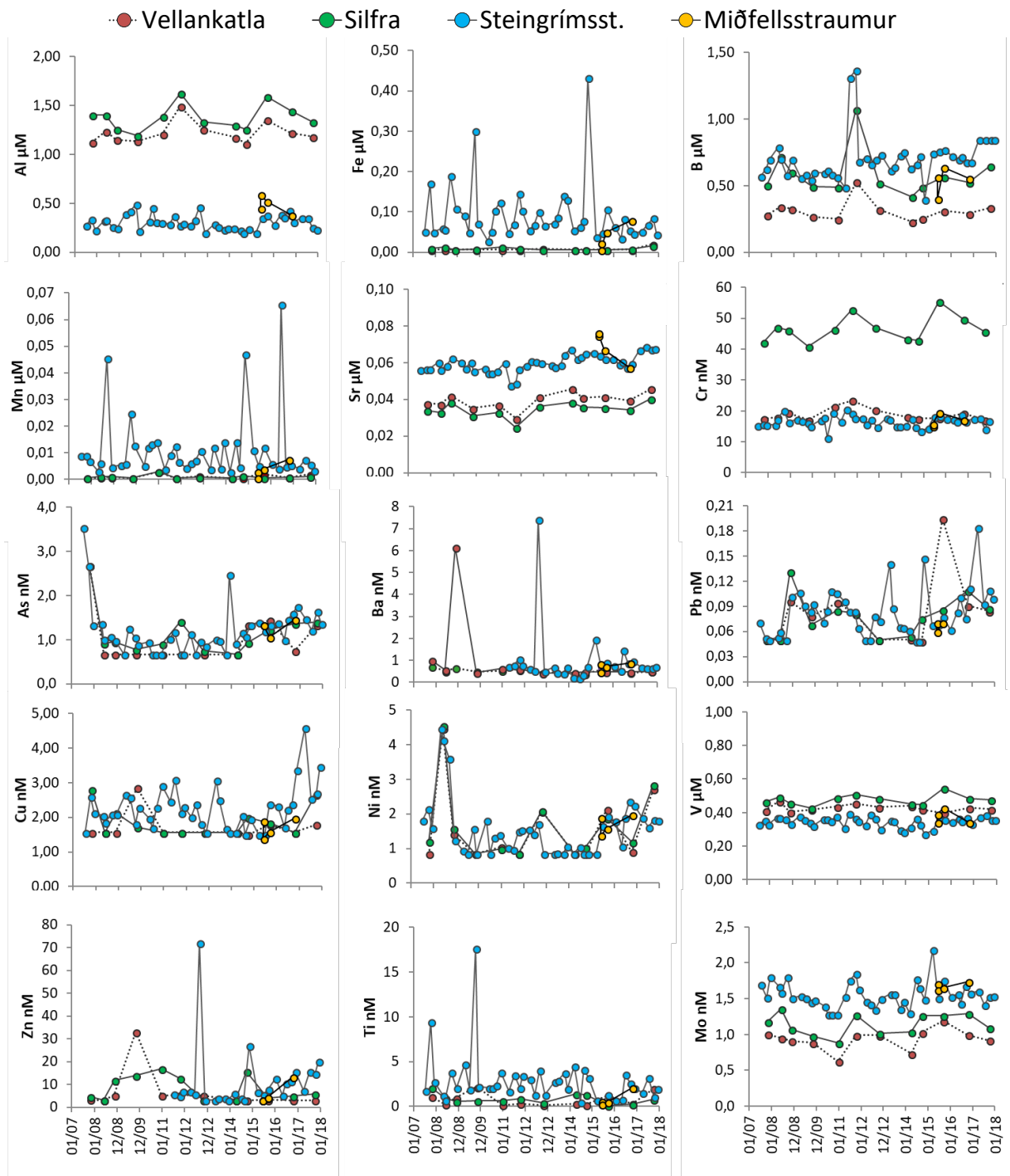
Mynd 7. Árstíðabundnar breytingar í styrk leystra snefilefna í inn- og útflæði Þingvallavatns. Söfnunarstaðirnir eru táknadír með mismunandi lit. Einingar eru í mikrómol/l ( \mu\text{M} ) og nanómol/l (nM).
