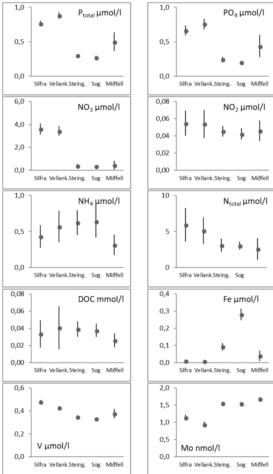
Mynd 11. Meðalstyrkur lífræns kolefnis og leystra næringarefna (með 95% öryggismörkum) úr innstreymi og útrennsli Þingvallavatns. Gögn úr Sogi við Þrastarlund frá 2007 til 2017 eru til samanburðar. Aðeins eru fjögur sýni úr Miðfellsstraumi.
