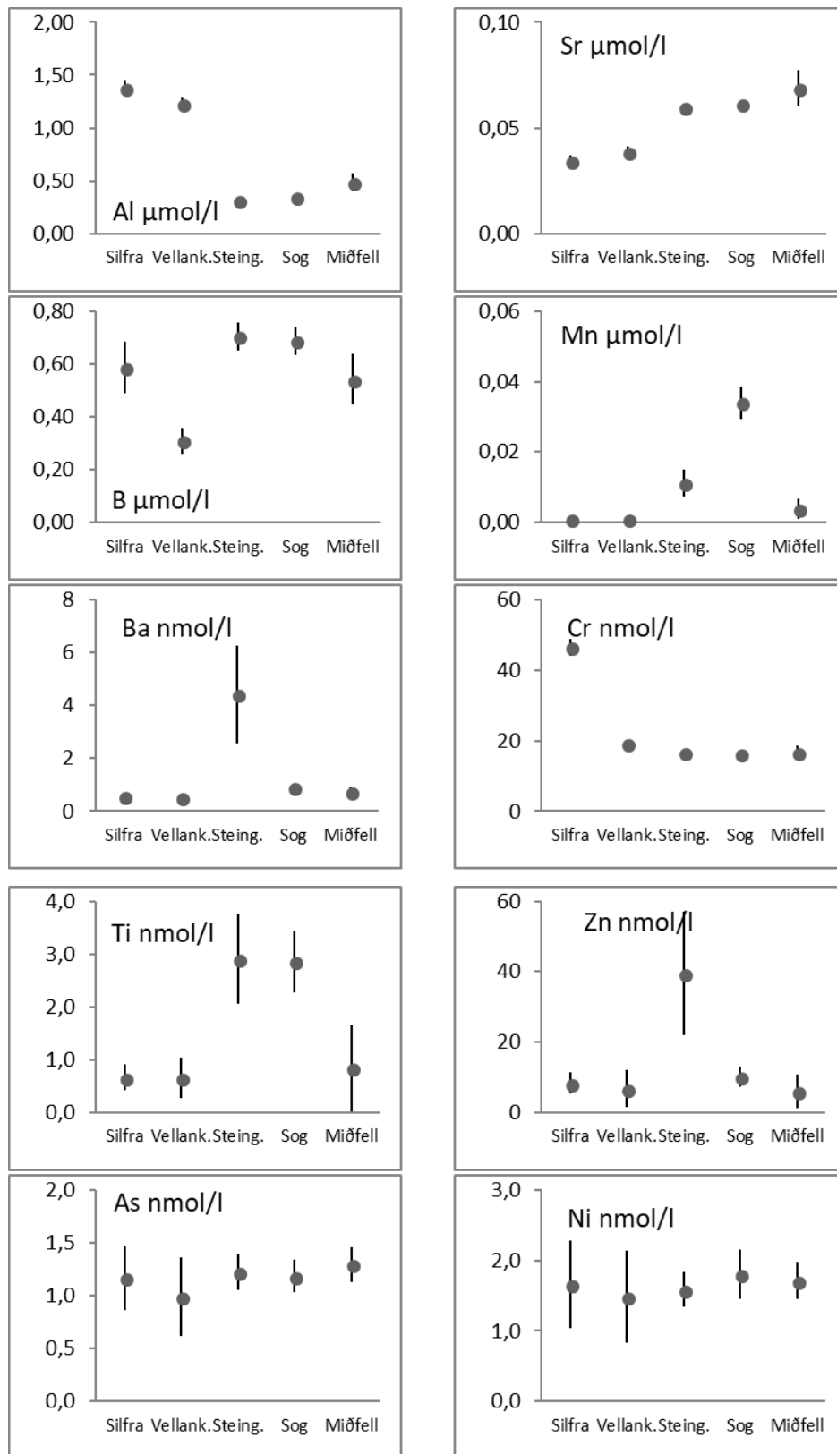
Mynd 12. Meðalstyrkur leystra þungmálma og annarra snefilefna (með 95% öryggismörkum) úr innstreymi og útrennsli Þingvallavatns. Gögn úr Sogi við Þrastarlund frá 2007 til 2017 eru til samanburðar. Aðeins eru fjögur sýni úr Miðfellsstraumi.
