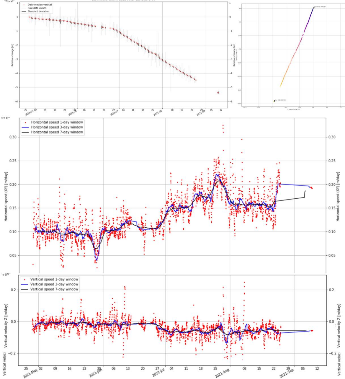
14. mynd. Efst: Færslur lóðrétt og lárétt á mælistað L05 mælt með landmælinga GPS (eftir á leiðrétt) frá lokum apríl til annarar viku september 2021. Miðja: hraði lárétrar hreyfingar og neðst hraði lóðrétrar hreyfingar, frá síðustu viku júní er stærstu hluti hreyfingarinnar vegna leysingar undan mastri GPS-tækisins.
