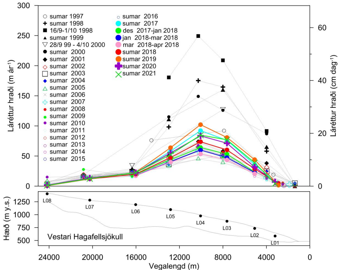
12. mynd. Þversnið niður miðjan Hagafellsjökul vestari (yfirborð 1997, punktar sýna yfirborðshæð 2020) og mældur láréttur yfirborðshraði í afkomumælistöðvum á því sniði haustin 1998 og 1999, sumurin 1997 til 2020 og 3 skipti veturinn 2017-18. Vel sést að sumarhraði 2017, 2018, 2019, 2020 og 2021 er aukinn, einkum 2017 og 2019, nærri L05, L04, L03 og L02 miðað við áratugin á undan, nú er væntanlega framhlaup í aðsigi.
